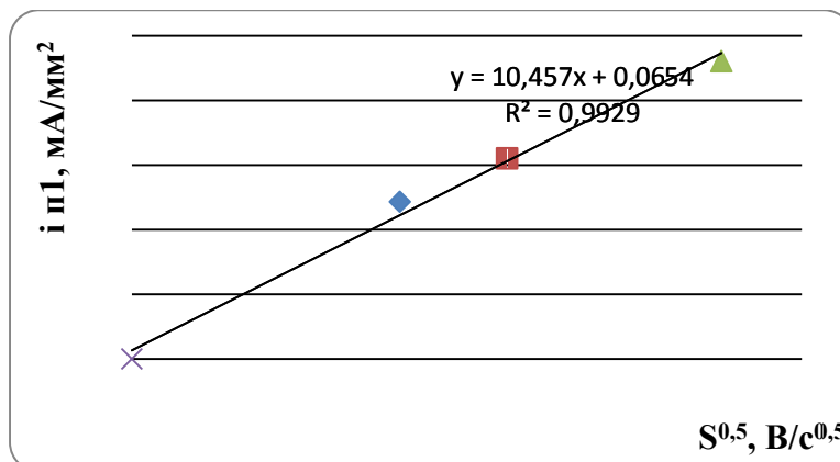
Рис.7. Зависимость плотности электрического тока пика ( i_{p1} , \text{mA/mm}^2 ) первой стадии анодного растворения олова от корня квадратного скорости развертки потенциала рабочего электрода ( S^{0.5} , (\text{V/s})^{0.5} )
